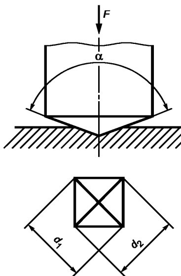
Рисунок 1 — Схема приложения нагрузки
